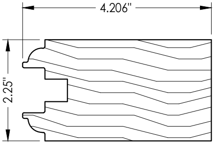
72 HINGE STILE Opaque Door
